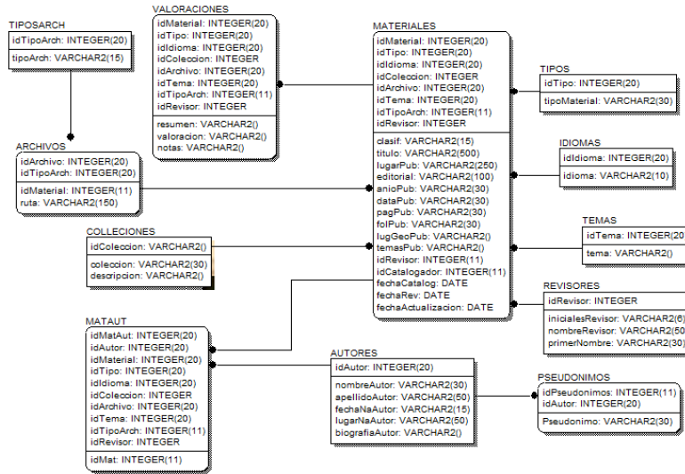
Figura 2. Diagrama relacional de la base de datos del sistema de captura.
